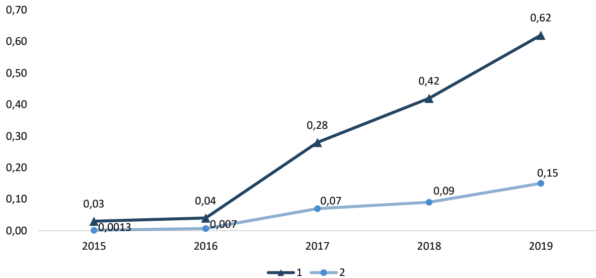
Рисунок 10.20 – Динамика доли ветровых и солнечных электростанций в структуре установленной мощности (1) и в выработке электрической энергии в ЕЭС Российской Федерации (2)
