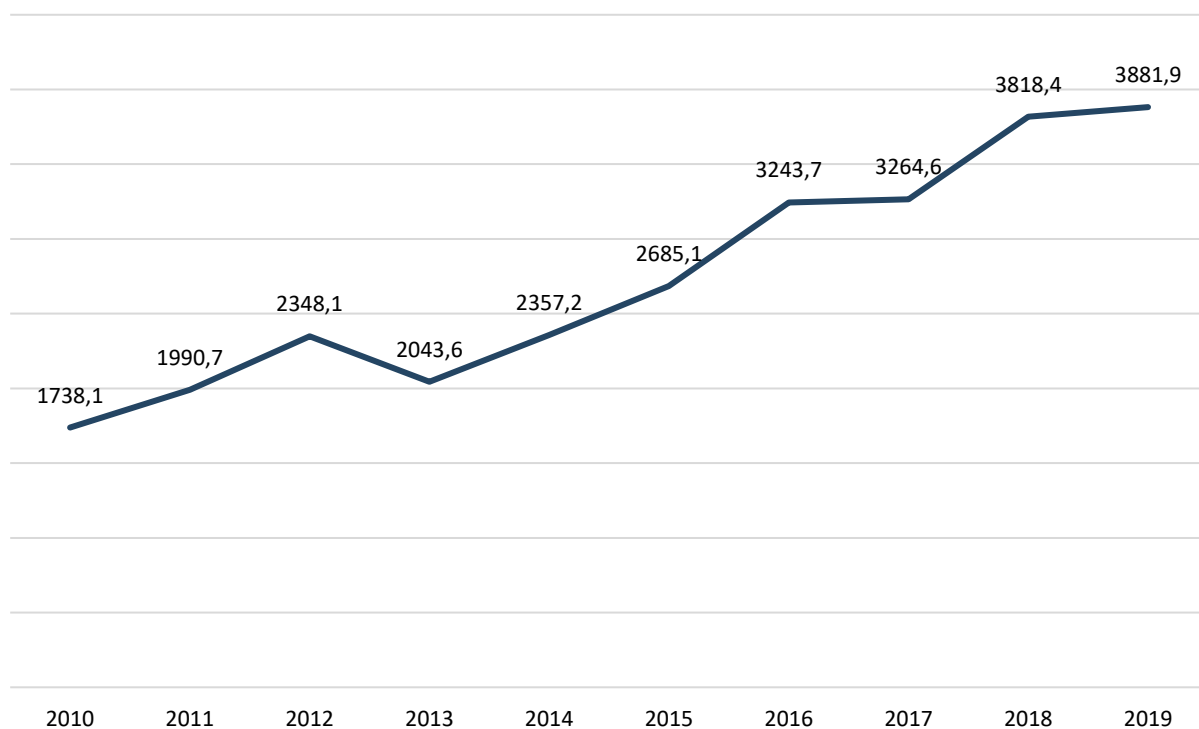
Рисунок 10.38 – Динамика утилизации и обезвреживания отходов производства и потребления в Российской Федерации 2010-2019 гг., млн т
