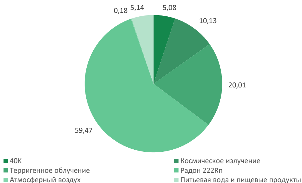
Рисунок 13.24 – Структура источников природного облучения населения по величине средней индивидуальной годовой эффективной дозы в период 2001-2018 г., %
