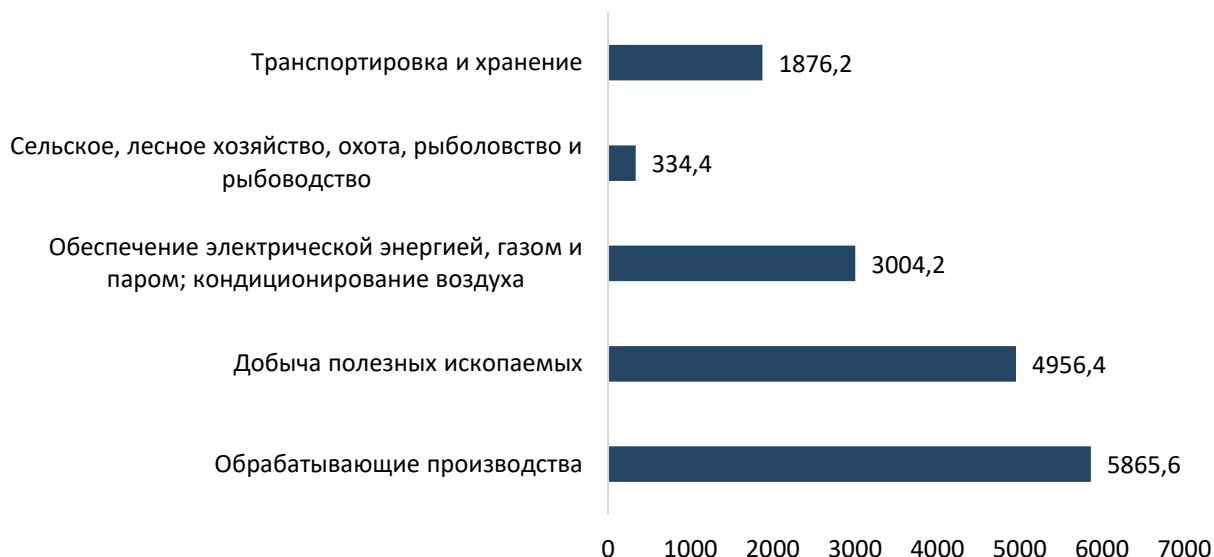
Рисунок 10.1 – Выбросы загрязняющих веществ в атмосферный воздух от стационарных источников по основным видам экономической деятельности в 2019 г., тыс. т
