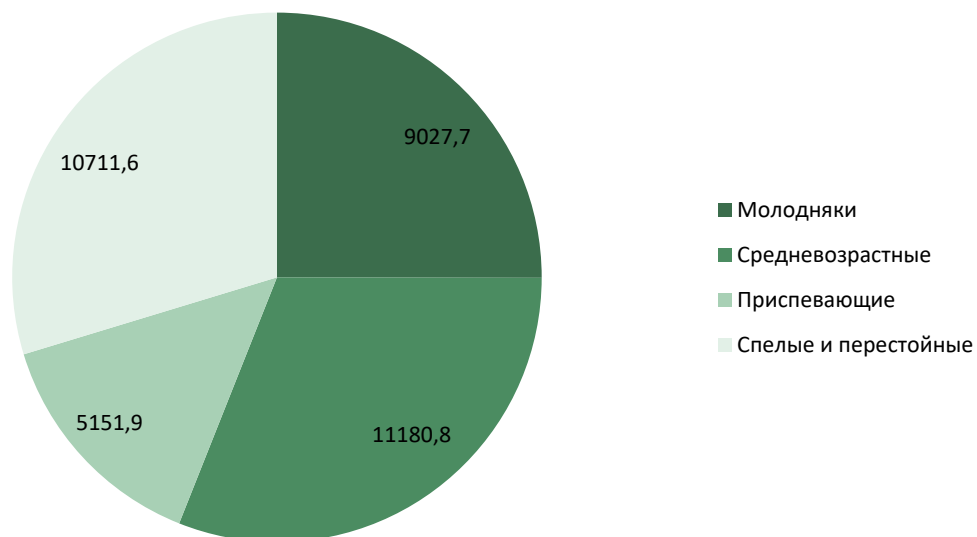
Рисунок 14.5.15 – Возрастная структура лесов Приволжского федерального округа в 2019 г., тыс. га
