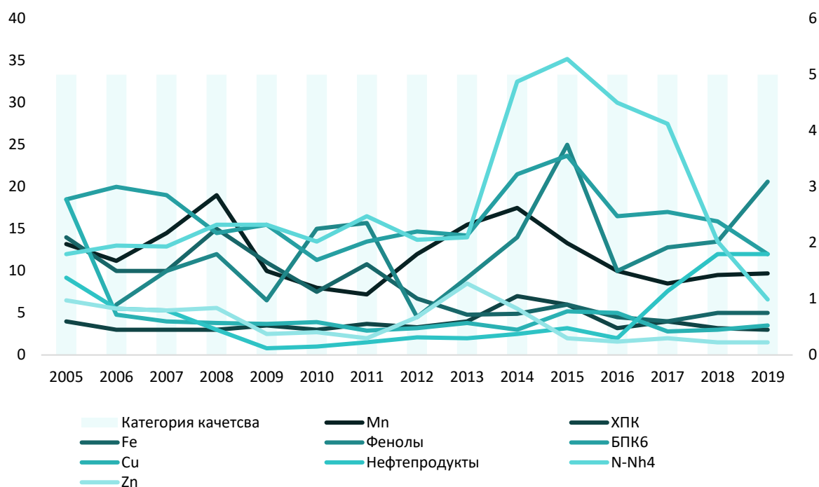
Рисунок 4.21 – Динамика среднегодового содержания основных загрязняющих веществ и качества воды р. Дачная в черте г. Арсеньев, 2005-2019 гг.
