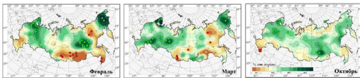
Рисунок 3.7 – Аномалии осадков в феврале, в марте, в октябре 2019 г.
