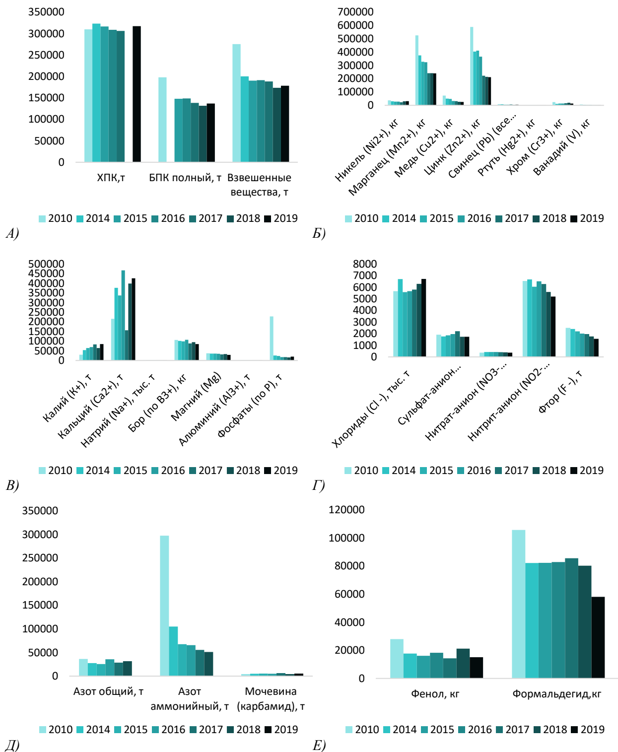
Рисунок 4.59 – Динамика сброса основных загрязняющих веществ в составе сточных вод в поверхностные природные водные объекты Российской Федерации, 2010-2019 гг.
