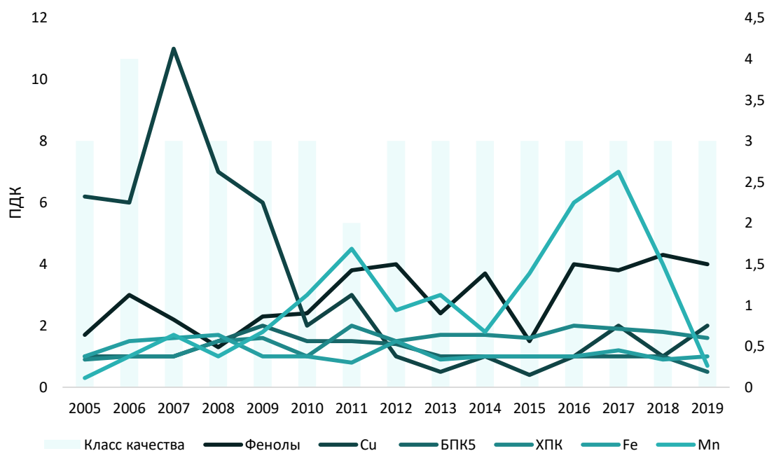
Рисунок 4.18 – Динамика среднегодовых концентрации отдельных загрязняющих веществ и показателе качества воды р. Лена, г. Якутск, 2004-2019 гг.
