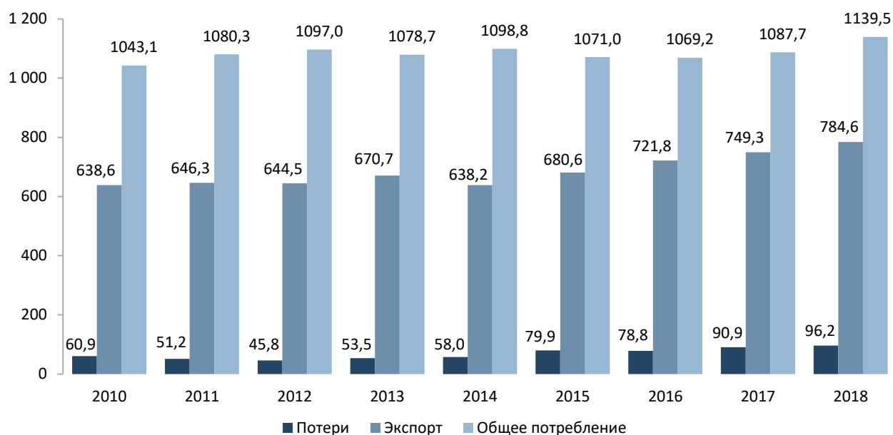
Рисунок 10.10 – Динамика структуры распределения энергоресурсов и их потерь при добыче, производстве и обогащении в Российской Федерации, 2010-2018 гг., млн т условного топлива
