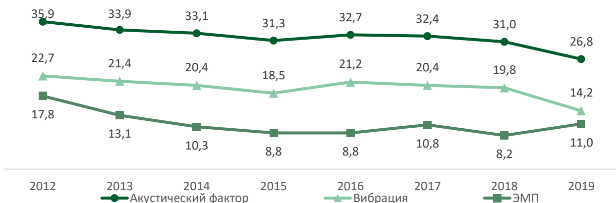
Рисунок 13.19 – Динамика удельного веса предприятий, воздействие которых не соответствует санитарным нормам по физическим факторам, 2012-2019 гг.
