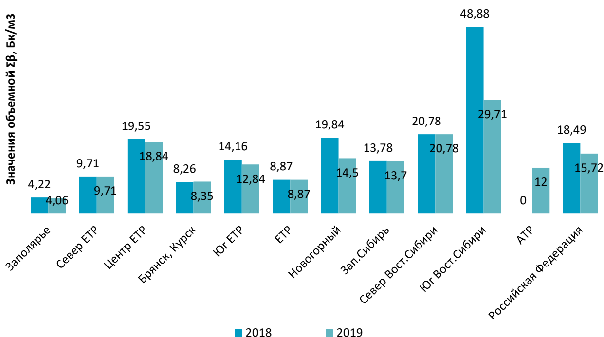
Рисунок 2.30 – Средние значения объемной \Sigma\beta в приземном слое атмосферы на территории Российской Федерации, 2018-2019 гг.
