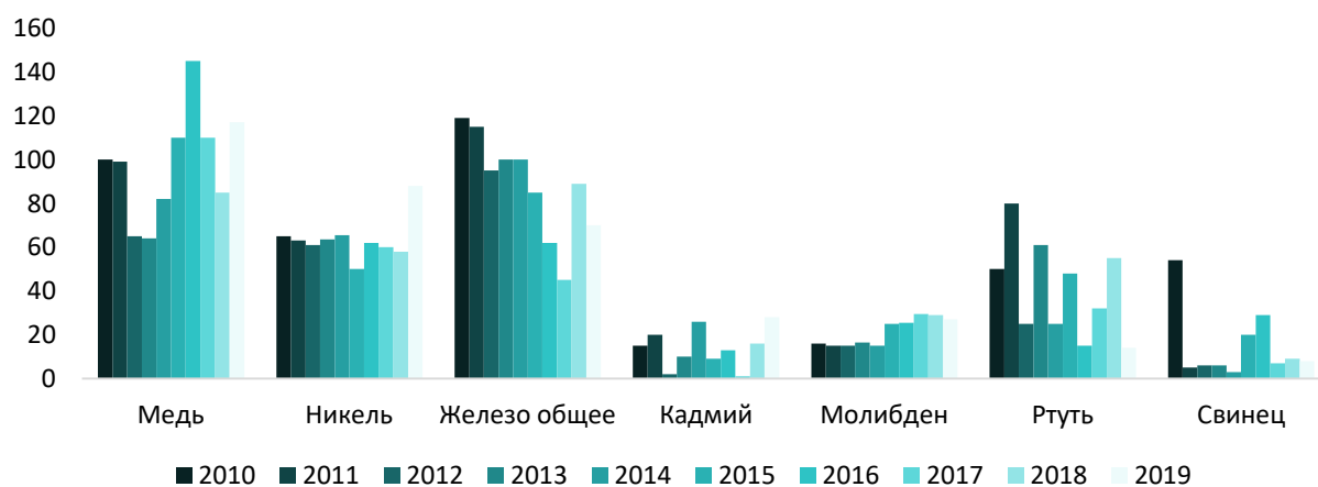
Рисунок 4.27 – Динамика случаев ВЗ и ЭВЗ поверхностных пресных вод некоторыми тяжелыми металлами, 2010-2019 гг.
