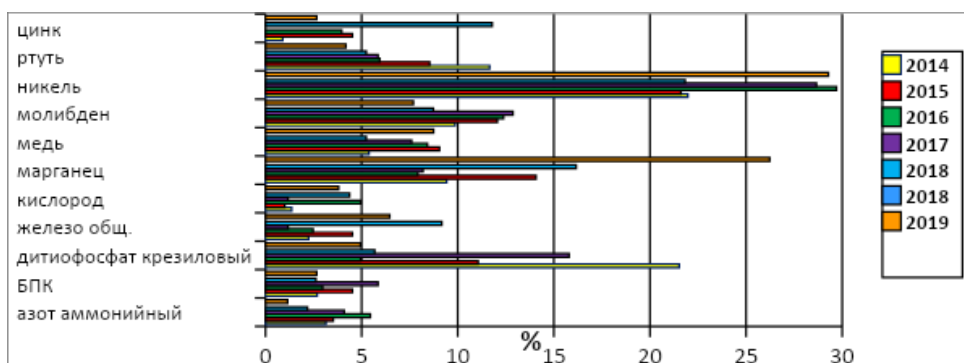
Рисунок 11.32 – Распределение числа случаев ВЗ и ЭВЗ по ингредиентам (в % от общего количества случаев ВЗ и ЭВЗ Арктической зоны Российской Федерации)
