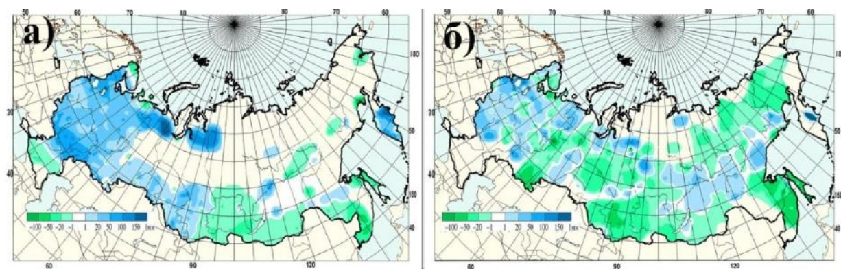
Рисунок 3.11 – Аномалии максимального запаса воды в снеге (мм) зимой 2018-2019 гг. (от среднемноголетних значений за период 1971-2000 гг.) в поле (а) и в лесу (б)
