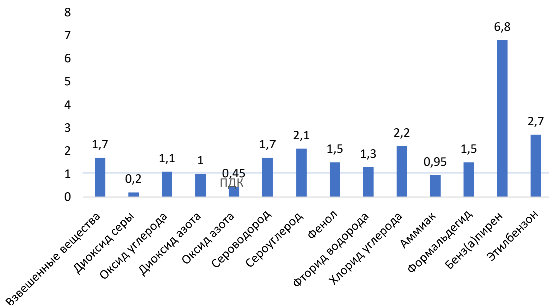
Рисунок 2.25 – Средние из максимальных концентраций примесей относительно ПДК в городах Российской Федерации, ПДК
