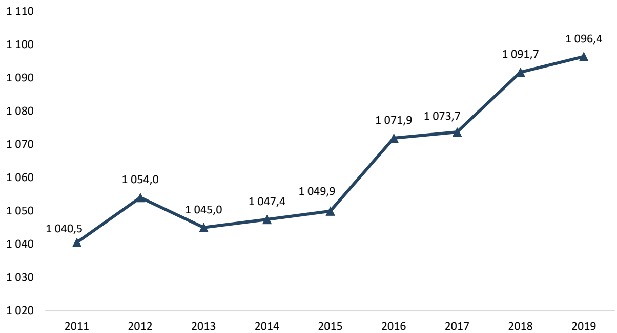
Рисунок 10.19 – Динамика выработки электроэнергии, 2011-2019 гг., млрд кВт*ч
