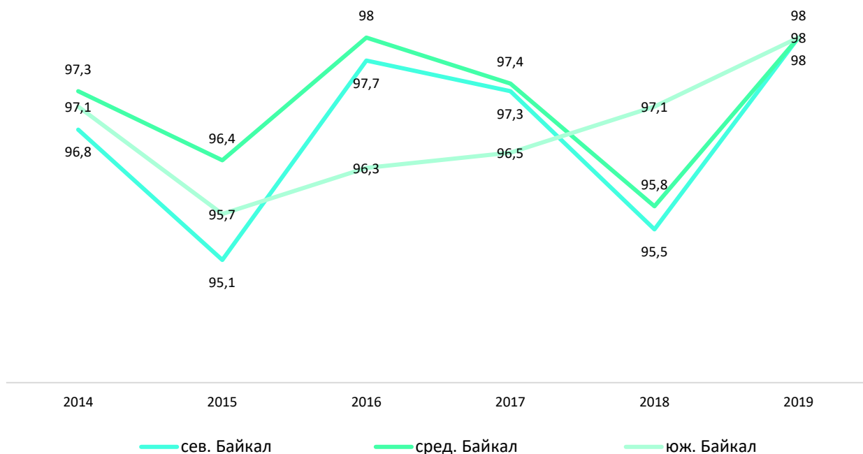
Рисунок 12.6 – Минерализация воды озера по котловинам продольного разреза, мг/л
