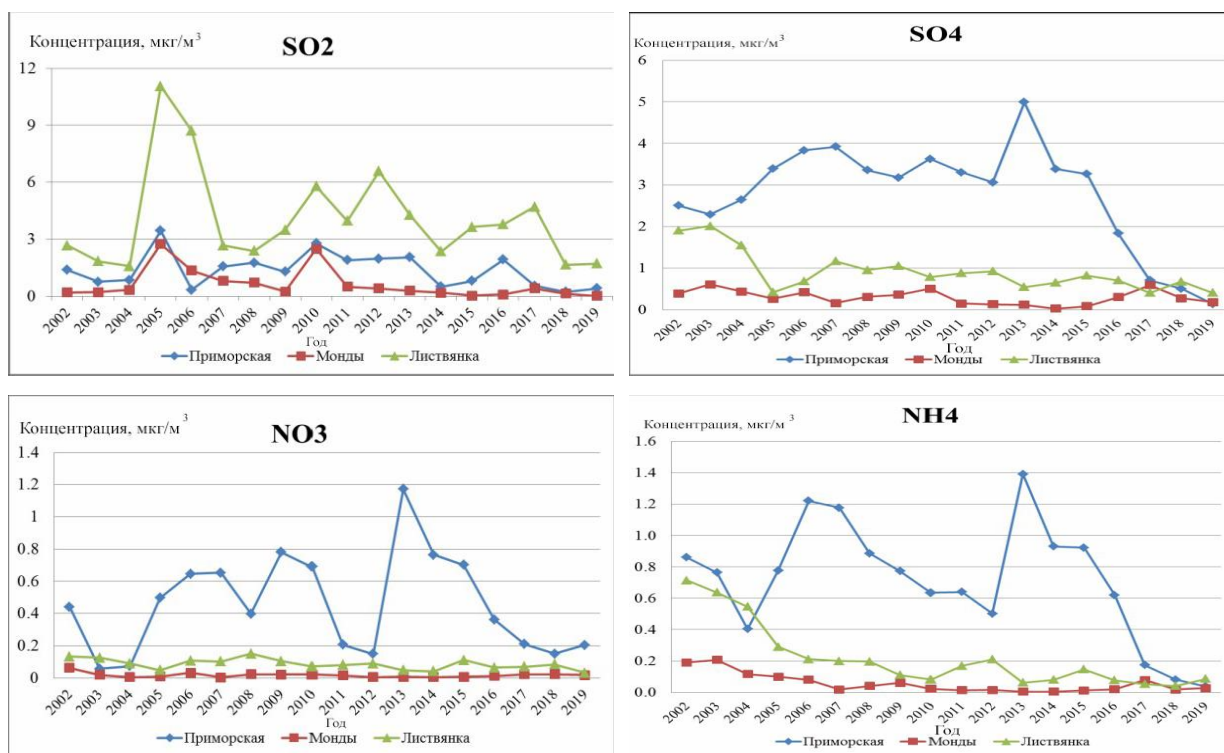
Рисунок 2.12 – Изменения средних годовых концентрации соединений серы (сверху) и азота (снизу) в воздухе на станциях ЕАНЕТ (мкг/м³)
