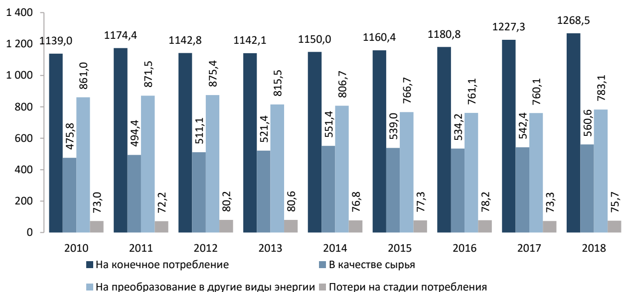
Рисунок 10.11 – Динамика структуры общего потребления энергоресурсов и их потерь на стадии потребления и транспортировки в Российской Федерации, 2010-2018 гг., млн т условного топлива
