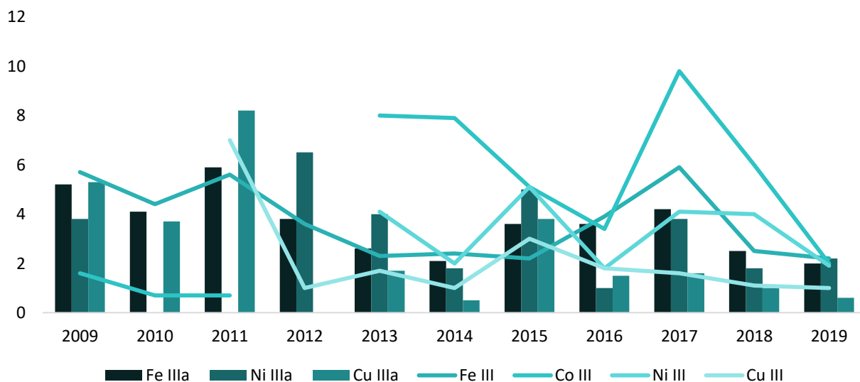
Рисунок 4.28 – Динамика среднегодовых концентраций концентрации железа (Fe), никеля (Ni) и меди (Cu) на разрезах III (Sec III) и IIIa (Sec IIIa) 2009-2019 гг.
