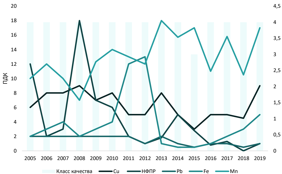
Рисунок 4.19 – Динамика среднегодовых концентраций отдельных ингредиентов и качества воды р. Колыма, п. Усть-Среднекан, 2005-2019 гг.
