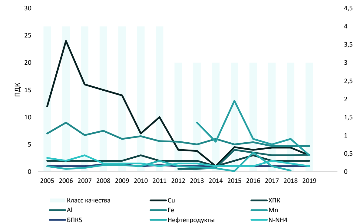
Рисунок 4.20 – Динамика среднегодового содержания основных загрязняющих веществ и качества воды в воде р. Амур, в пункте г. Амурск, 2005-2019 гг.
