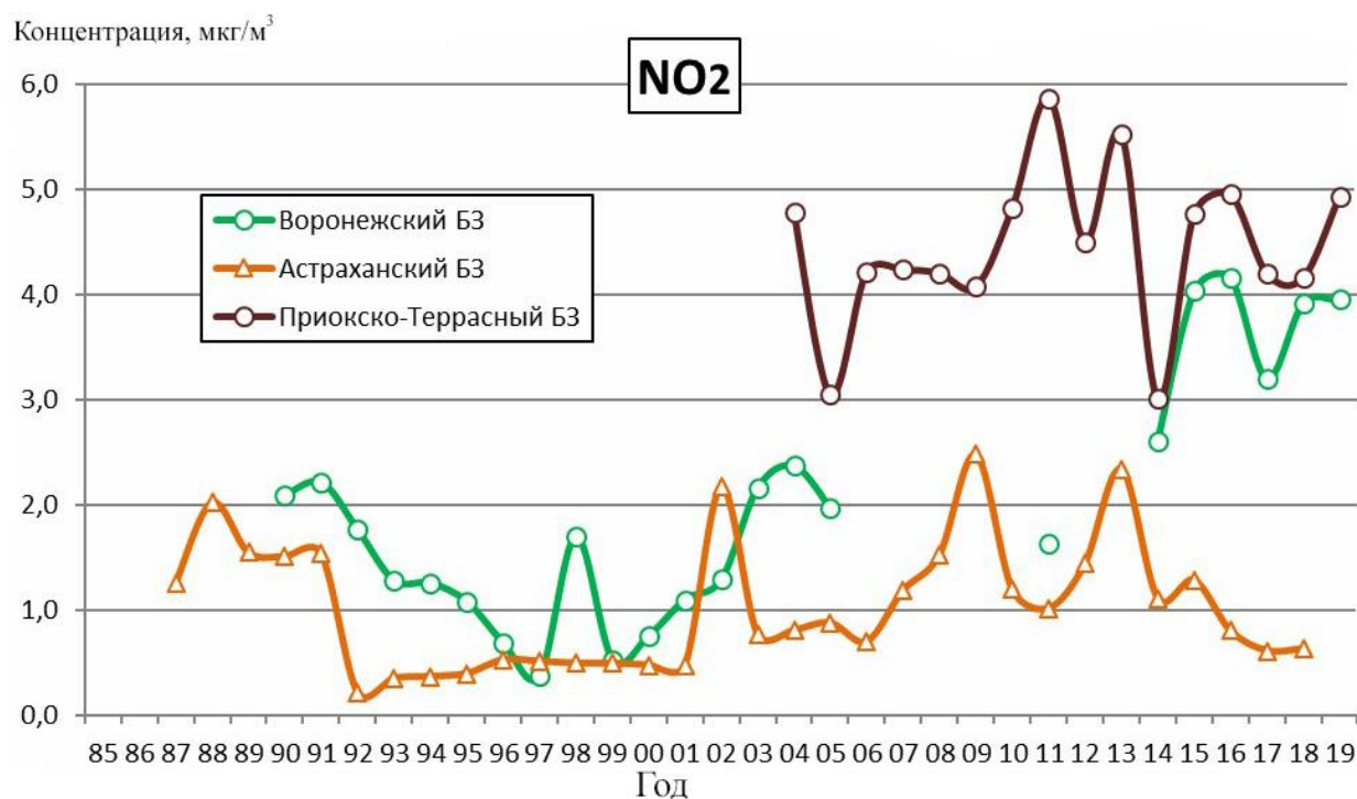
Рисунок 2.5 – Динамика фонового содержания диоксида азота в атмосферном воздухе фоновых районов, 1987-2019 гг., нг/м 3
