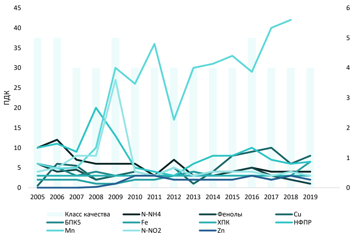
Рисунок 4.16 – Динамика среднегодовых концентраций отдельных загрязняющих веществ и показателей качества воды р. Каменка, 2005-2019 гг.
