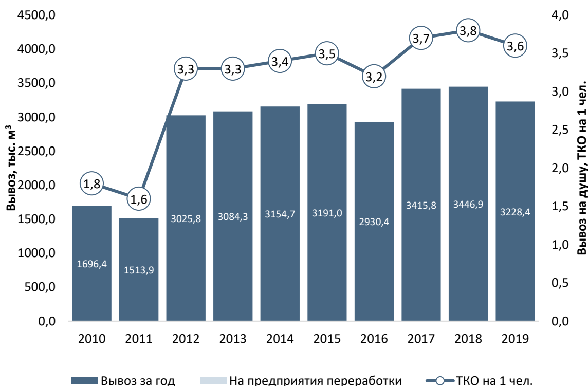
Рисунок 14.5.64 – Вывоз твердых коммунальных отходов, 2010-2019 гг.
