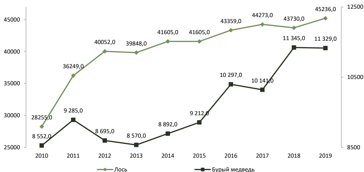
Рисунок 14.2.29 – Динамика численности лося и бурого медведя, 2010-2019 гг., особей Источник: составлено авторами
