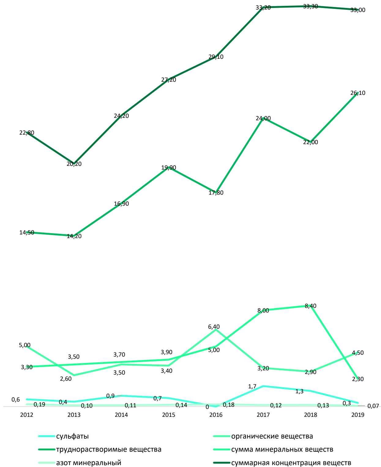
Рисунок 12.5 – Динамика поступления химических веществ из атмосферы на ст. Хужир, тонн/год на км 2
