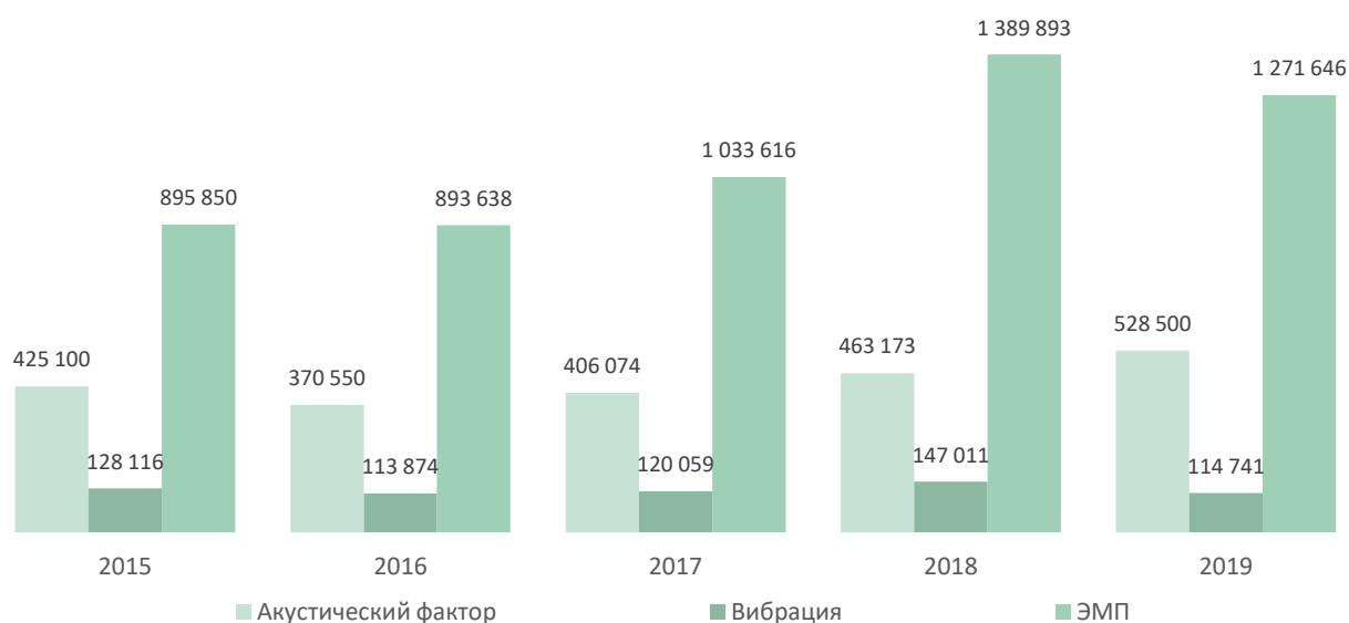
Рисунок 13.20 – Динамика общего количества выполненных измерений, результаты которых не соответствуют санитарным нормам по приоритетным физическим факторам, 2015-2019 гг.
