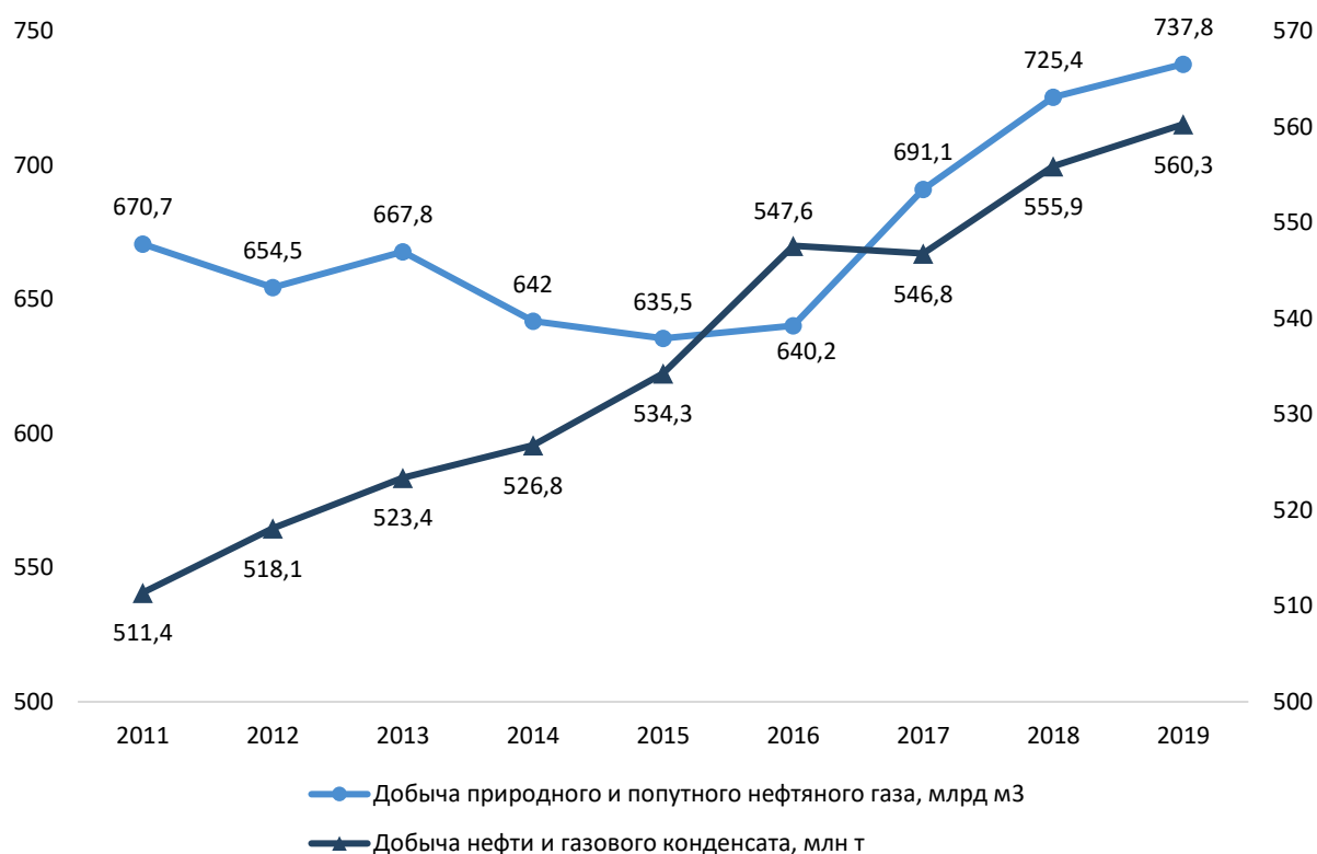
Рисунок 10.17 – Динамика добычи природного и попутного нефтяного газа, нефти и газового конденсата, 2011-2019 гг.
