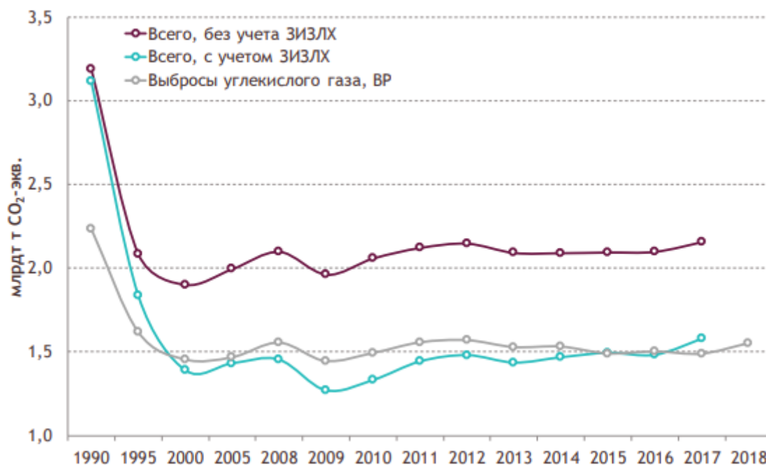
Рисунок 3.24 – Совокупные антропогенные выбросы парниковых газов в Российской Федерации, млрд т CO 2 -экв., 1990-2018 гг.
