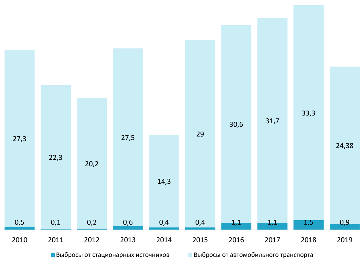
Рисунок 14.4.33 – Динамика выбросов загрязняющих веществ в атмосферный воздух в 2010-2019 гг., тыс. т
