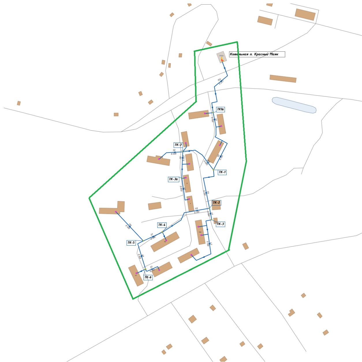
Рисунок 3. Зона действия котельной п. Красный Маяк
